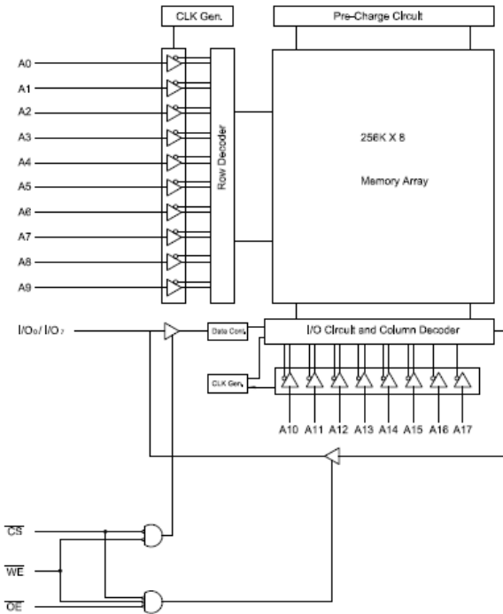
CS18FS2048(3/W) – (256k x 8)
